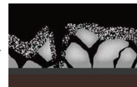
アルミ系酸化生成物が充填される前に犠牲防食作用が働かなくなり、腐食が進行してしまう。
